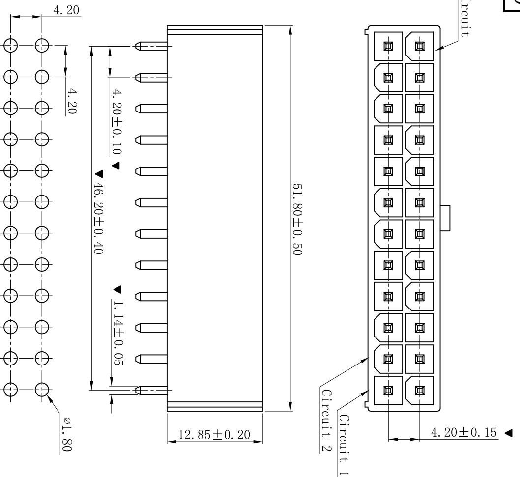
P.C.B LAYOUT
