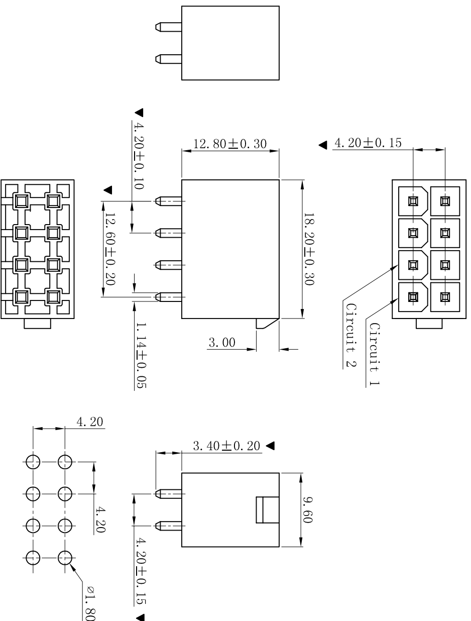
P.C.B LAYOUT
