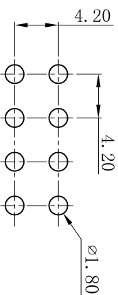
P.C.B LAYOUT
