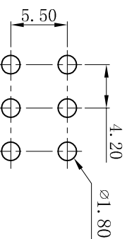
P.C.B LAYOUT
