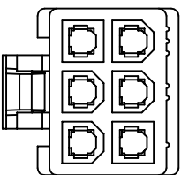
2方4圆孔位 (PCI)
