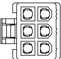
3方3圆孔位 (3F3V)
