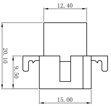
H3682-03P H3682NE-03P
