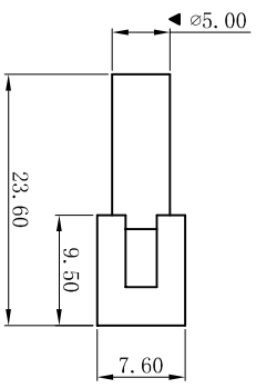
H3682-01P
