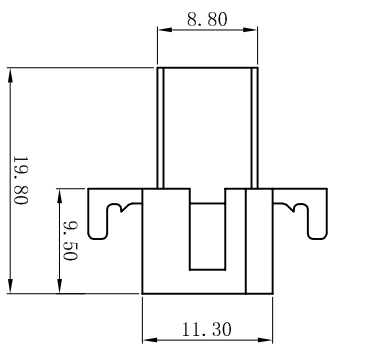
H3682-02P H3682NE-02P
