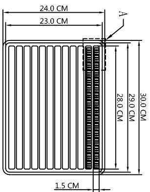
吸塑盘下盖(12格)
